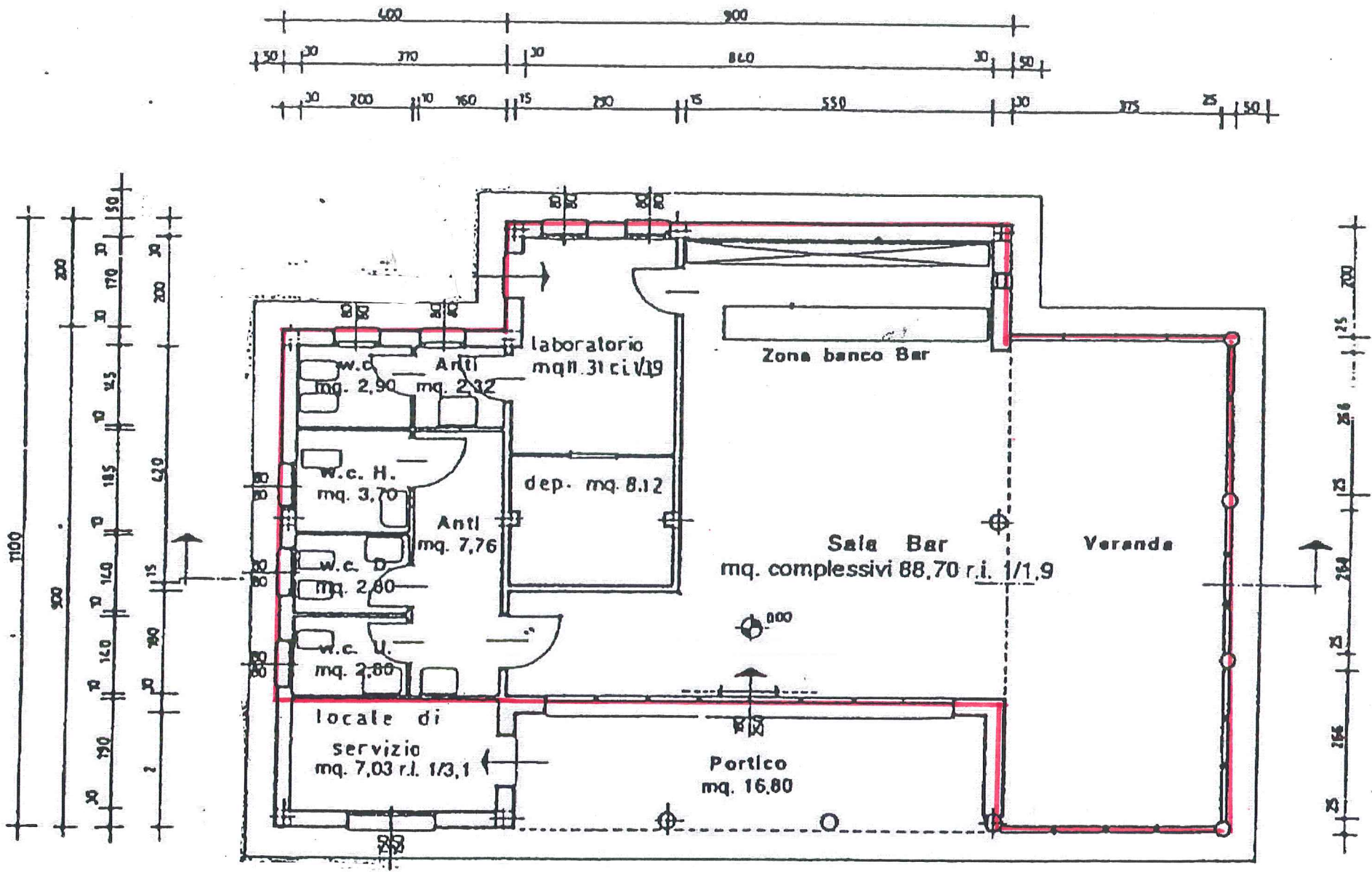
PIANTA PIANO TERRA - 1:200 - PALAZZINA EST
