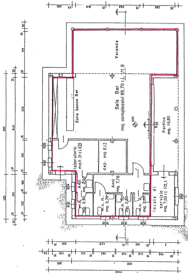
PIANTA PIANO TERRA - 1:200 - PALAZZINA EST
